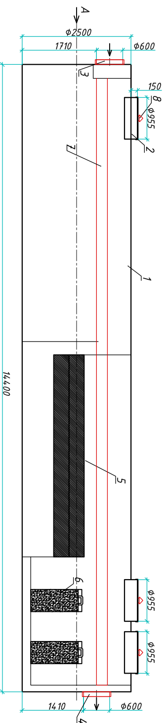
Разрез 1-1
