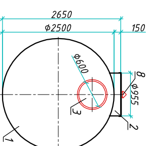
Вид А
